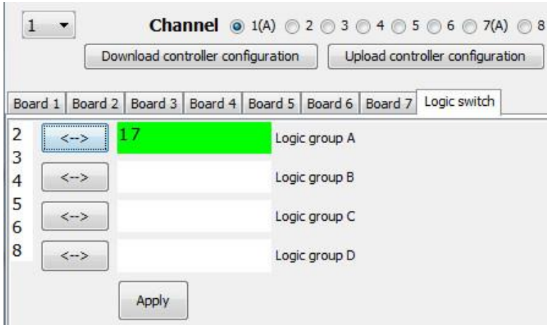
Logic group 1A: TST8801 1, Kanavat 1 ja 7 (=LSW1 ja hälytin)
